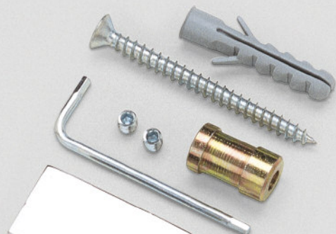
Art. M3000 Portatubo Ø 16 mm con accessori. Tube support for Ø 16 mm with fittings. Palier de tube pour Ø 16 mm avec accessoires.
