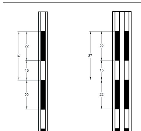
Dimensione passo / spacing 37 mm
